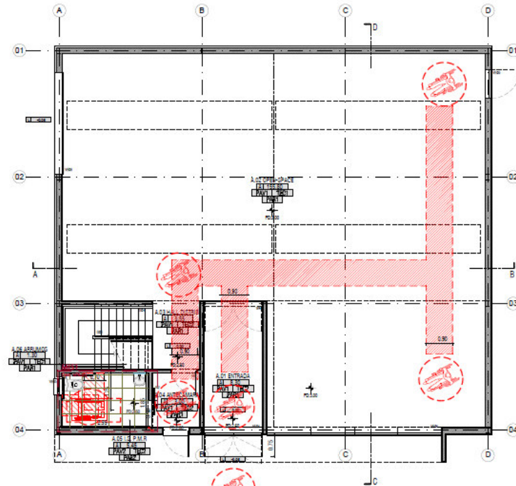
PLANO DE ACESSIBILIDADES ESC. 1/100
